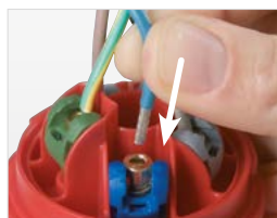
1) Insert wire
