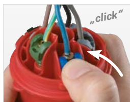
2) Close terminal
